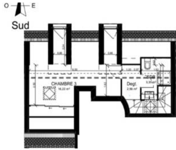
Niveau Combles
